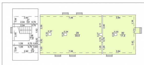
Третий этаж S=50.8 m2
