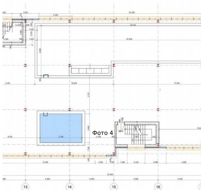
План-схема (эскипия) 1-го этажа на отм. +0,000
