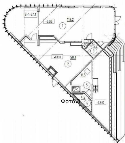
ПЛАН 1 этаж
