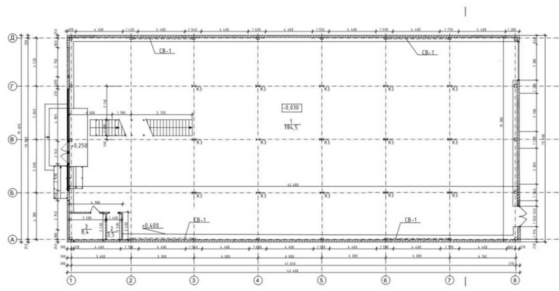
План первого этажа
